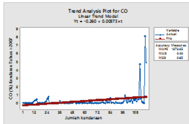
Gambar 5. Trend Analysis Plot For Variabel Bebas CO Mobil di Atas Tahun 2007
