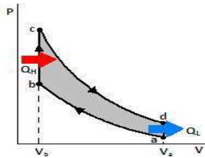
Gambar 1. Siklus Motor Bensin
