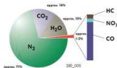
Gambar 2. Komposisi gas buang motor bensin
